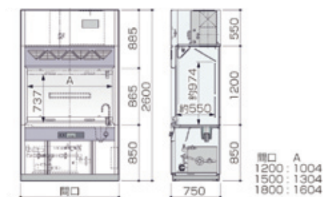
尺寸图 (mm)
